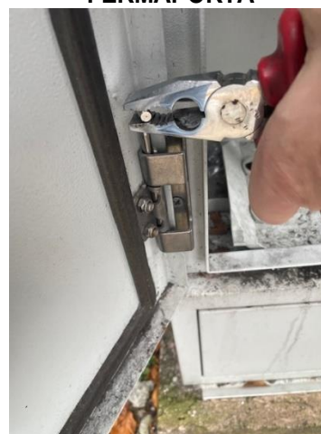
3 - TOGLIERE PERNO CERNIERE E SPOSTARE LA PORTA
