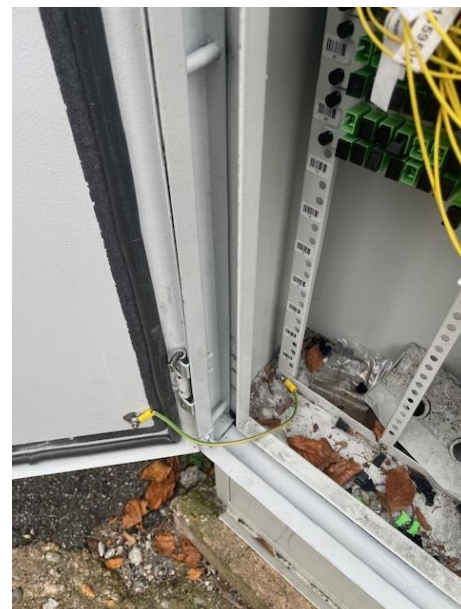
7 – COLLEGARE IL CAVO DI MESSA A TERRA PRESENTE SULLA PORTA
